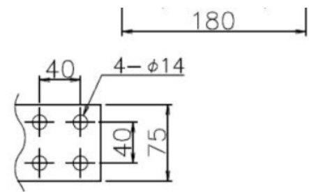
一次端子 P'ry Terminal 1200~1500A 端子厚さ 10mm
