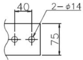
一次端子 P'ry Terminal ~1000A 端子厚さ 6mm
